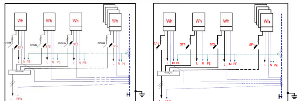
6 paveikslas. Įvadinės apskaitos spintos skirtos įrengti šešioms ir daugiau trifazių elektros skaitiklių principinė elektros schema
