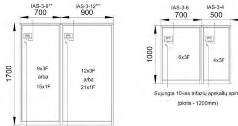
Sujungta 21-nių trifazių arba 36-ių vienfazių apskaitų spinta (plois 1600mm)
