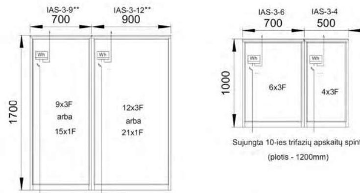
Sujungta 21-rių trifazių arba 36-ių vienfazių apskaitų spinta (plois 1600mm)
